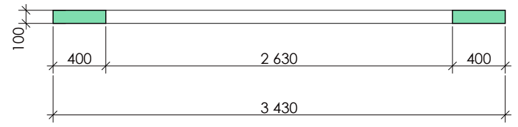
Конструкция ГКЛ №3
