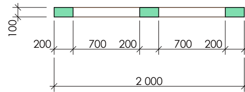
Конструкция ГКЛ №2
